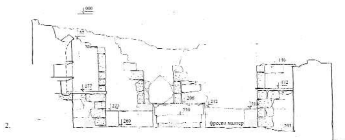
Пресеж источниј део цркве и западни изглед
