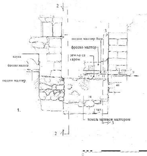
Сонда 7. ЈИ угао зидова Пресеци 1-1
